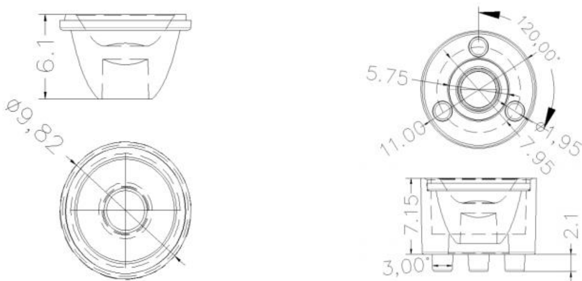
透镜外形尺寸 Len profile dimensions
