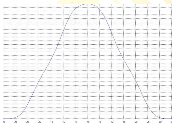
光曲线-直角坐标 Light distribution curve-right-angle coordinates
