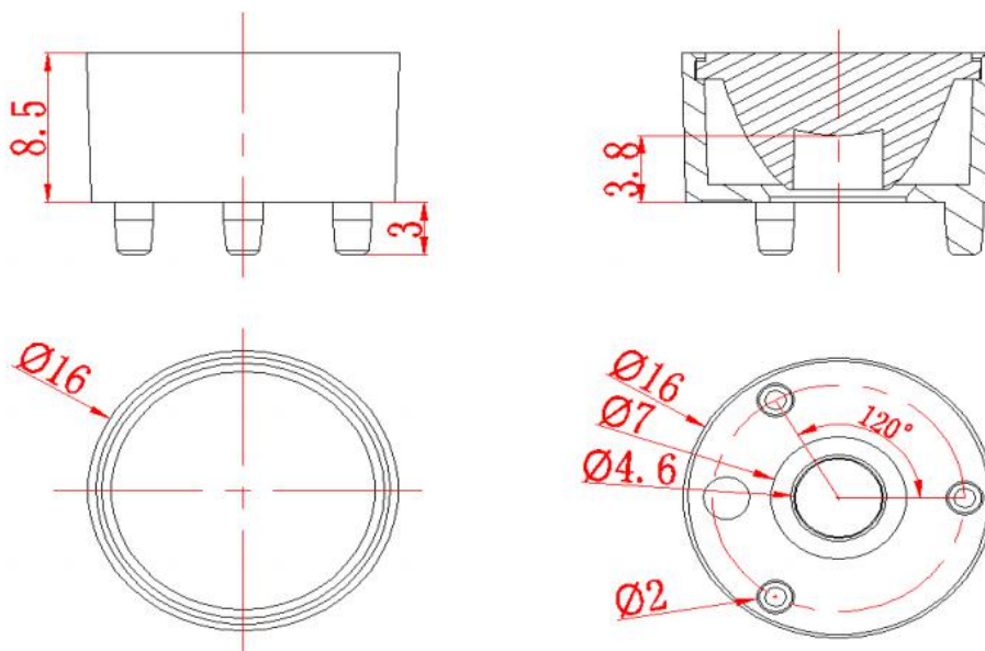
透镜外形尺寸 Len profile dimensions
