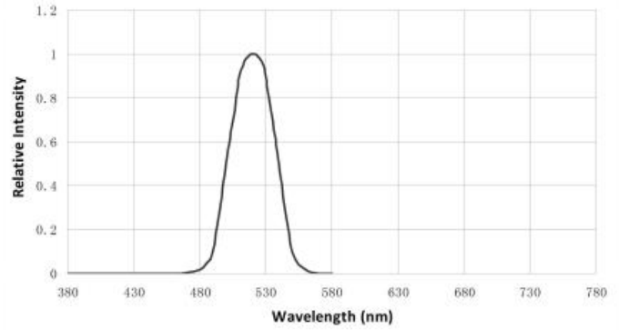
光谱分布特性曲线 Spectrum Distribution ( T_a=25^\circ\text{C} )
